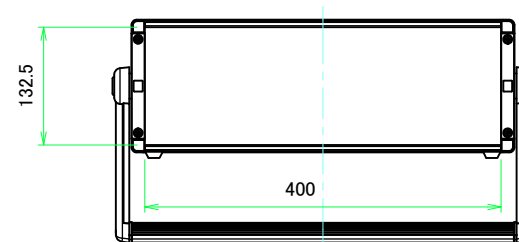
サイドフレーム2 / Side frame2
