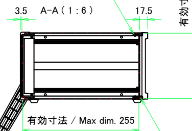
リアフレーム1 / Rear frame1
