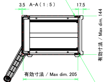
リアフレーム1 / Rear frame1
