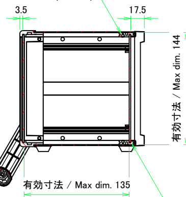
リアフレーム1 / Rear frame1
