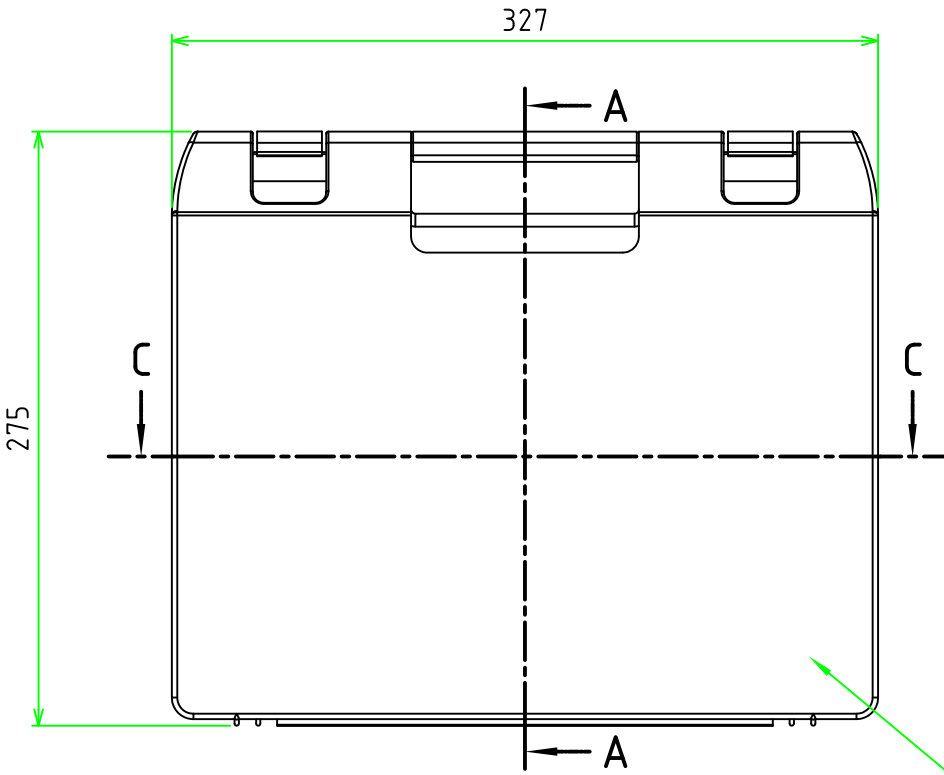
ベース側 / Base
