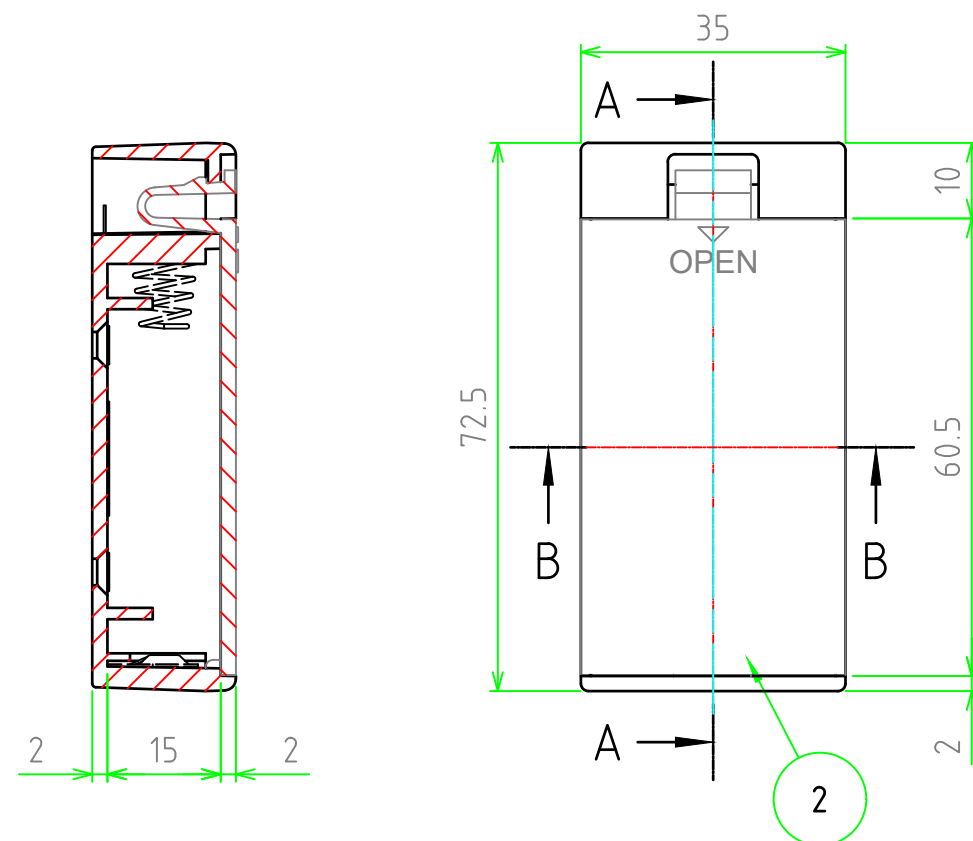
A-A断面図
