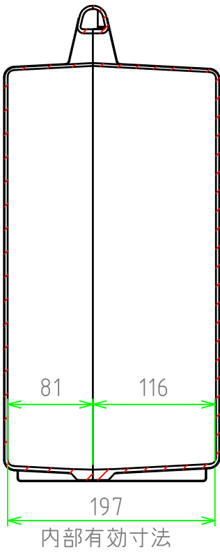
A-A 断面図
