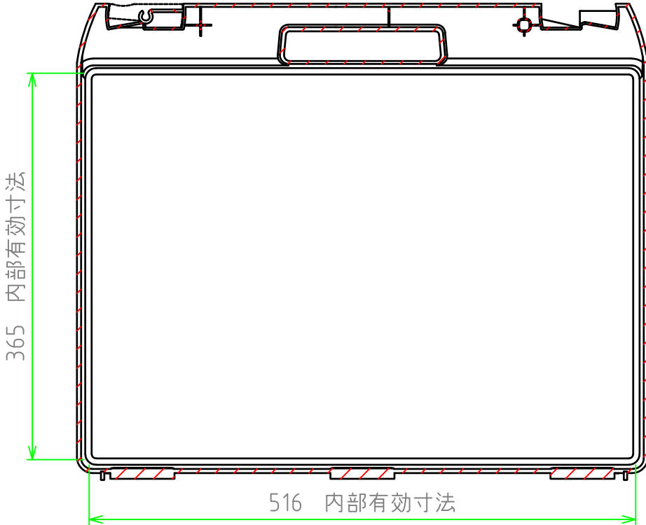
B-B 断面図
