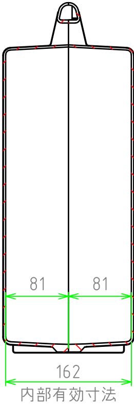
A-A 断面図
