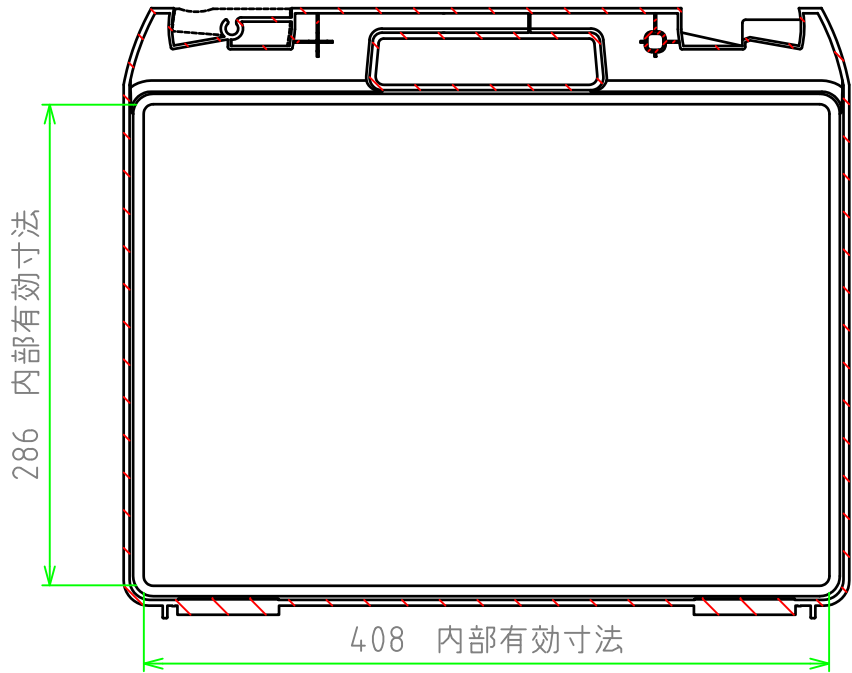
B-B 断面図
