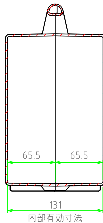
A-A 断面図
