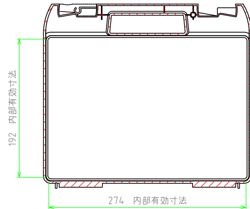
B-B 断面図
