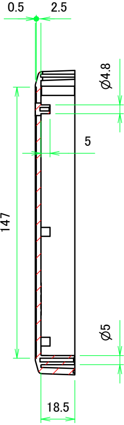
C-C ( 1 : 2 )
