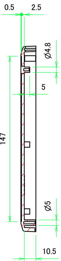
C-C ( 1 : 2 )
