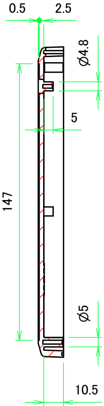
C-C ( 1 : 2 )
