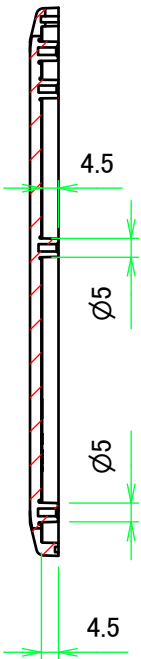
C-C ( 1 : 2 )
