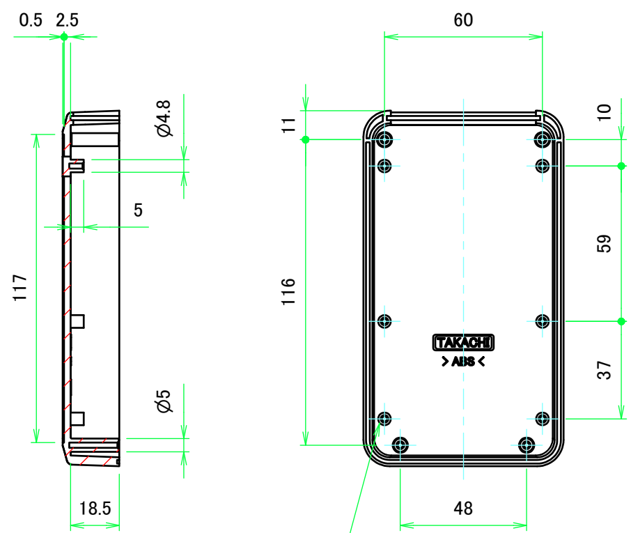
C-C ( 1 : 2 )
