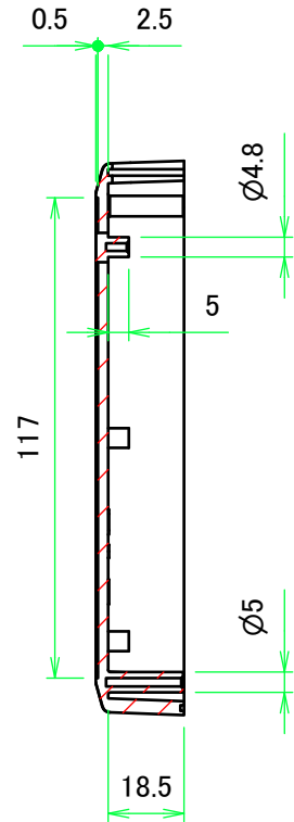
C-C ( 1 : 2 )
