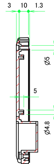
E-E ( 1 : 2 )
