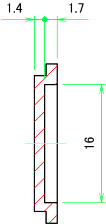
G-G ( 2 : 1 )
