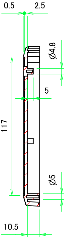
C-C ( 1 : 2 )
