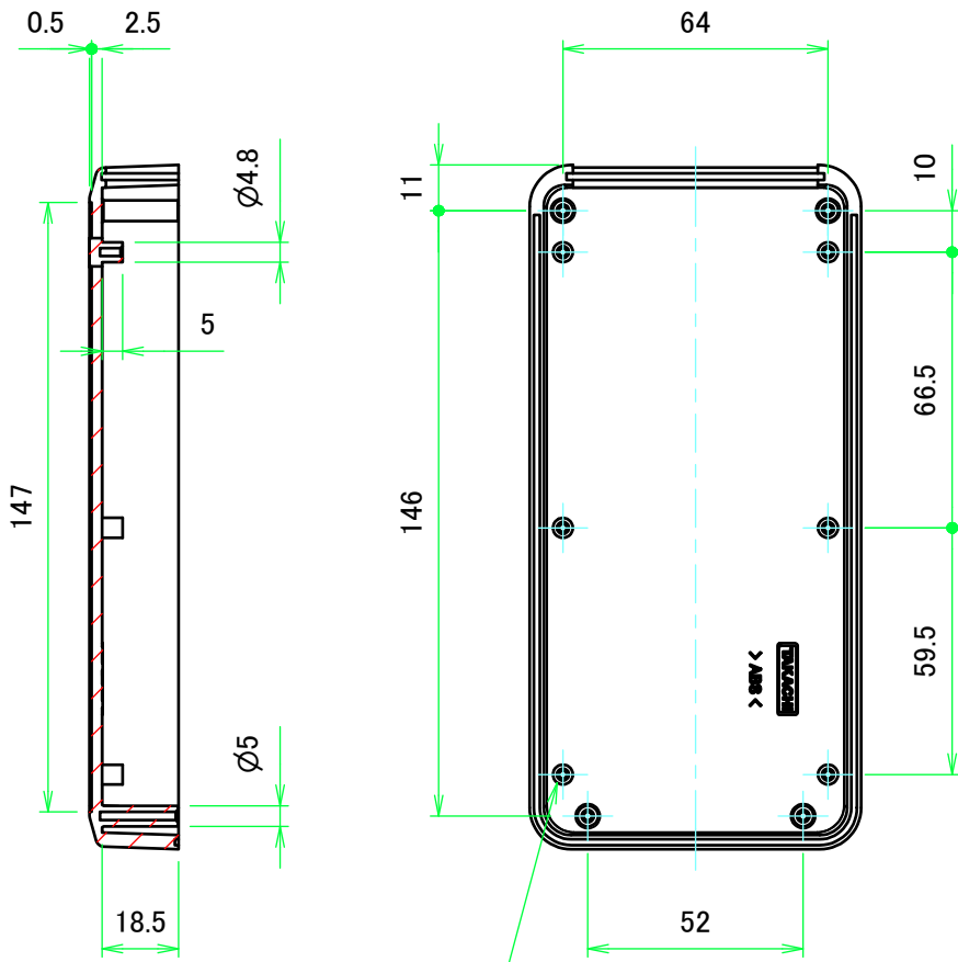
C-C ( 1 : 2 )
