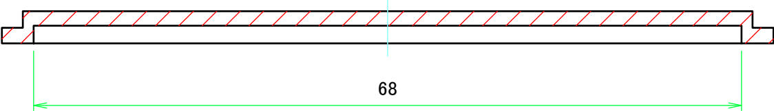
H-H ( 2 : 1 )
