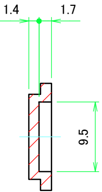
G-G ( 2 : 1 )
