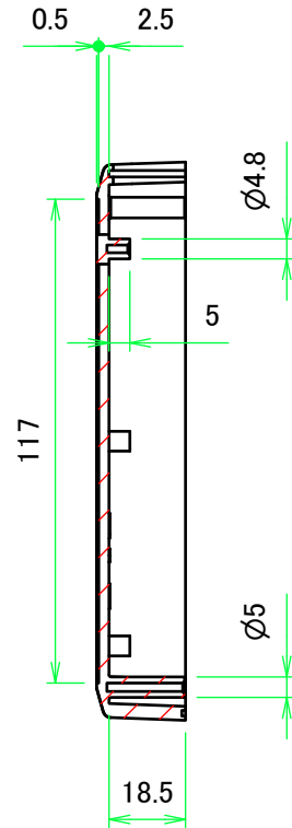
C-C ( 1 : 2 )
