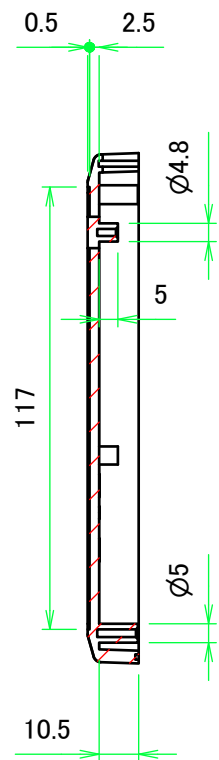
C-C ( 1 : 2 )
