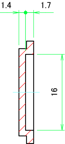
G-G ( 2 : 1 )
