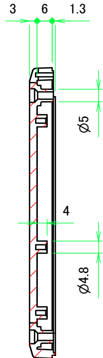
E-E ( 1 : 1.5 )
