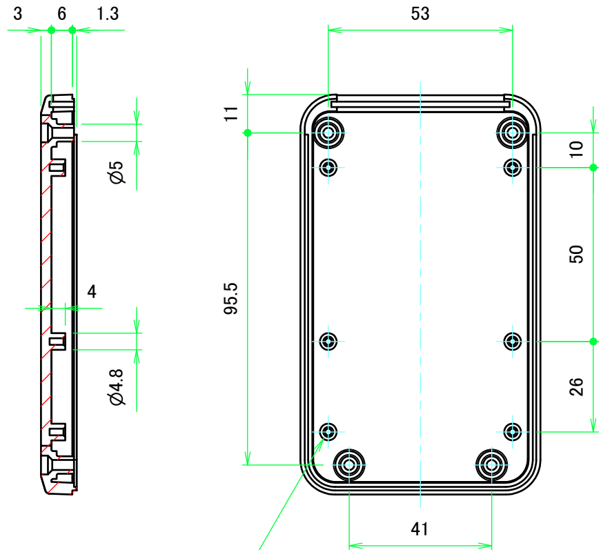
E-E ( 1 : 1.5 )
