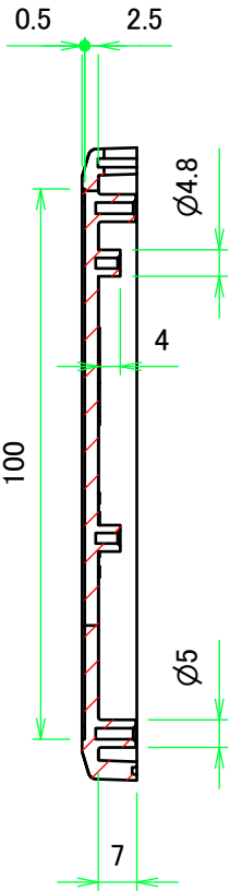
C-C ( 1 : 1.5 )
