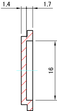
G-G ( 2 : 1 )
