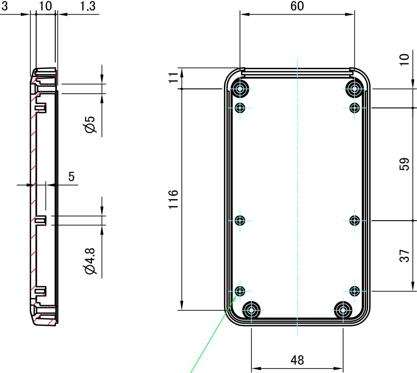
6-M2.3用基板取付ボス 6-M2.3 Boss
