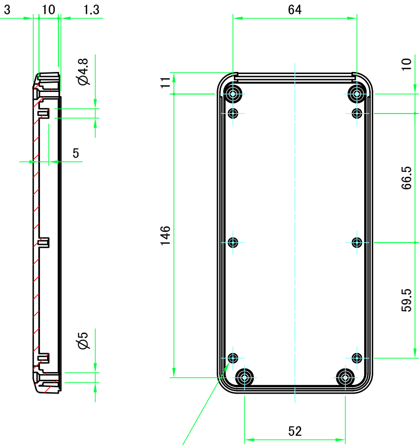
6-M2.3用基板取付ボス 6-M2.3 Boss
