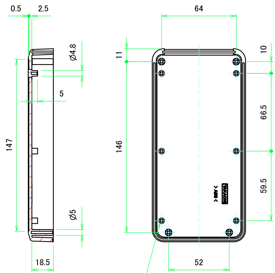
C-C ( 1 : 2 )
