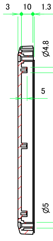
E-E ( 1 : 2 )
