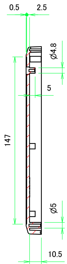
C-C ( 1 : 2 )
