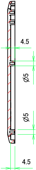
C-C (1:2)
