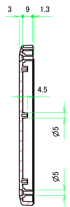
E-E ( 1 : 2 )
