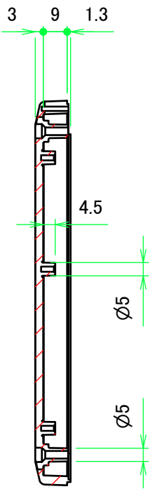
E-E ( 1 : 2 )
