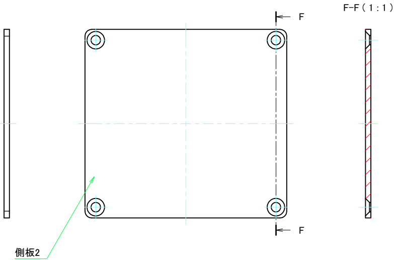
側板2
