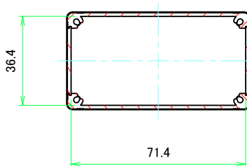
A-A (1:1.5)
