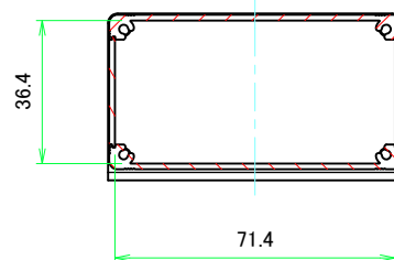
A-A (1:1.5)
