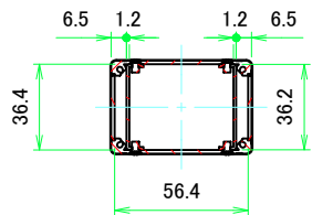
A-A (1:2.5)
