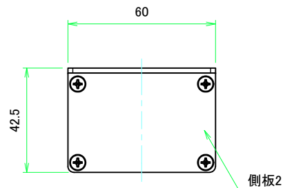
側板2
