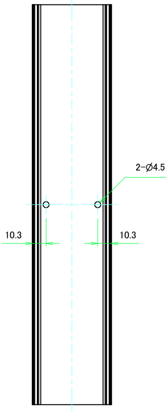
カバーフレーム1 (内視)
