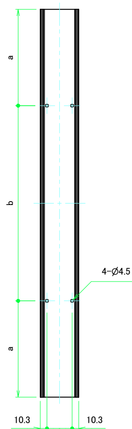
カバーフレーム1(内視)
