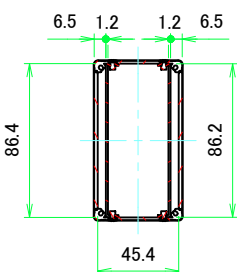
A-A (1:3)
