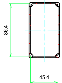
A-A (1:2.5)
