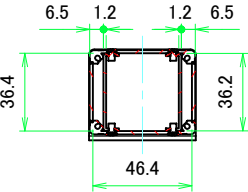
A-A ( 1 : 2.5 )
