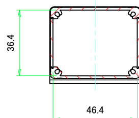
A-A (1:1.5)
