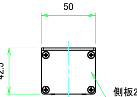
側板2
