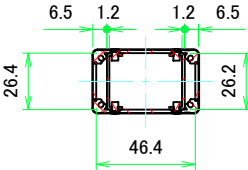
A-A ( 1 : 2.5 )
