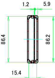
A-A (1:3)
