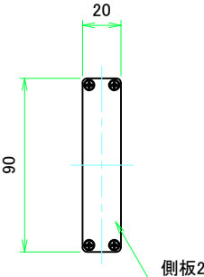
側板2
