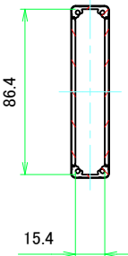
A-A (1:2.5)
