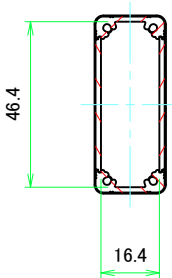
A-A ( 1 : 1.5 )
