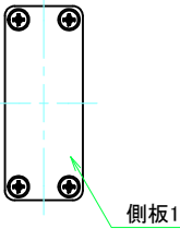
A-A ( 1 : 1.5 )
