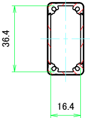
A-A ( 1 : 1.5 )
