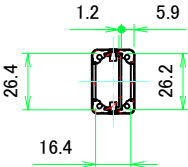
A-A ( 1 : 2.5 )
