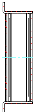
B-B ( 1 : 1.5 )
