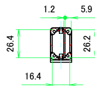
A-A (1:2.5)
