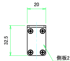
側板2
