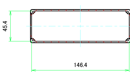
A-A ( 1 : 2.5 )
