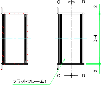
B-B ( 1 : 2.5 )
