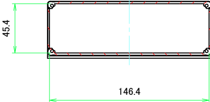
A-A ( 1 : 2.5 )
