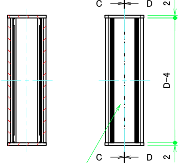
フラットフレーム1
