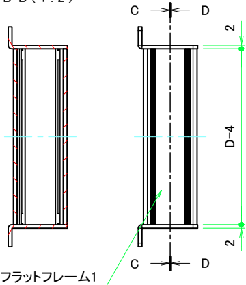
B-B (1:2)
